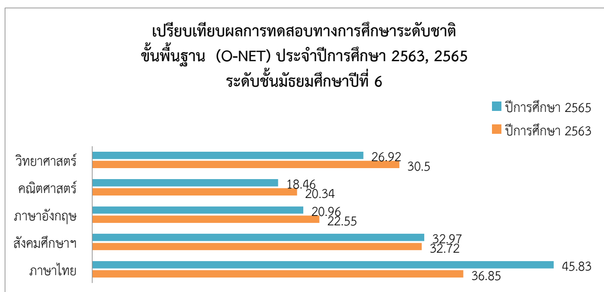
แผนภาพ 7 เปรียบเทียบผลการทดสอบทางการศึกษาระดับชาติขั้นพื้นฐาน (O-NET) ประจำปีการศึกษา 2563, 2565 ชั้นมัธยมศึกษาปีที่ 6
