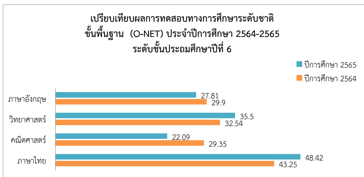
แผนภาพ 5 เปรียบเทียบผลการทดสอบทางการศึกษาระดับชาติด้านพื้นฐาน (O-NET) ประจำปีการศึกษา 2564-2565 ระดับชั้นประถมศึกษาปีที่ 6
