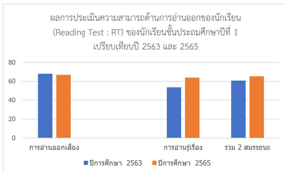
แผนภาพ 3 เปรียบเทียบผลการประเมินความสามารถด้านการอ่านออกของนักเรียน (Reading Test : RT) ของนักเรียนชั้นประถมศึกษาปีที่ 1 ปีการศึกษา 2563 และ 2565
