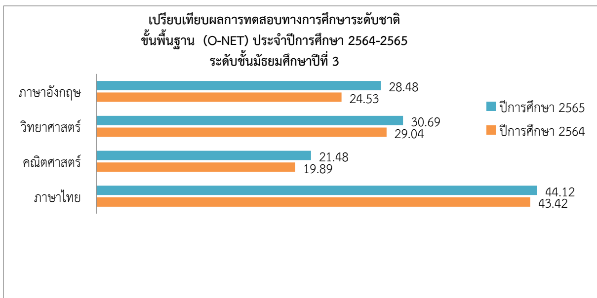
แผนภาพ 6 เปรียบเทียบผลการทดสอบทางการศึกษาระดับชาติด้านขั้นพื้นฐาน (O-NET) ประจำปีการศึกษา 2564-2565 ระดับชั้นมัธยมศึกษาปีที่ 3
